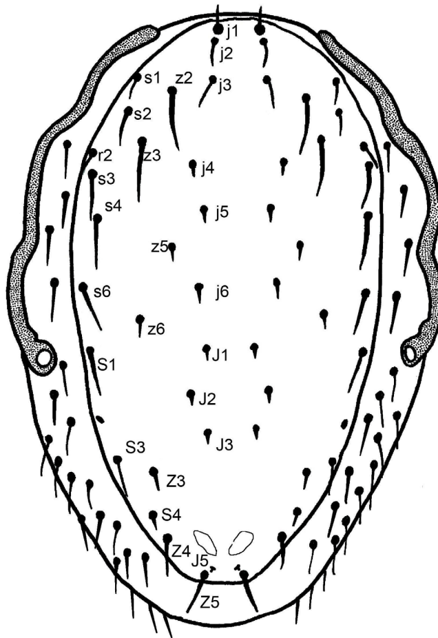
Fig. 1. Macronyssus stanyukovichi Orlova et Zhigalin, 2015, male, dorsal idiosoma. Scale bar 100 \mu m.
