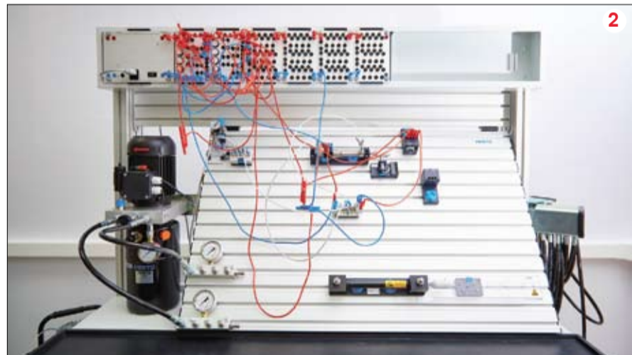
Учебный стенд «Гидропневмопривод» (Фото 2)
