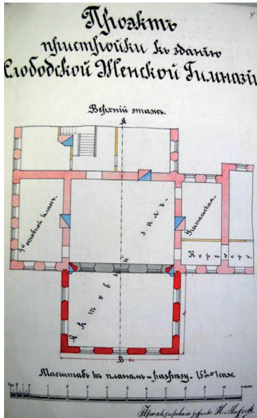
Рис. 9. Проект пристройки к зданию Слободской женской гимназии 1913 г. Ф. 583, оп. 536, ед. хр. 153
