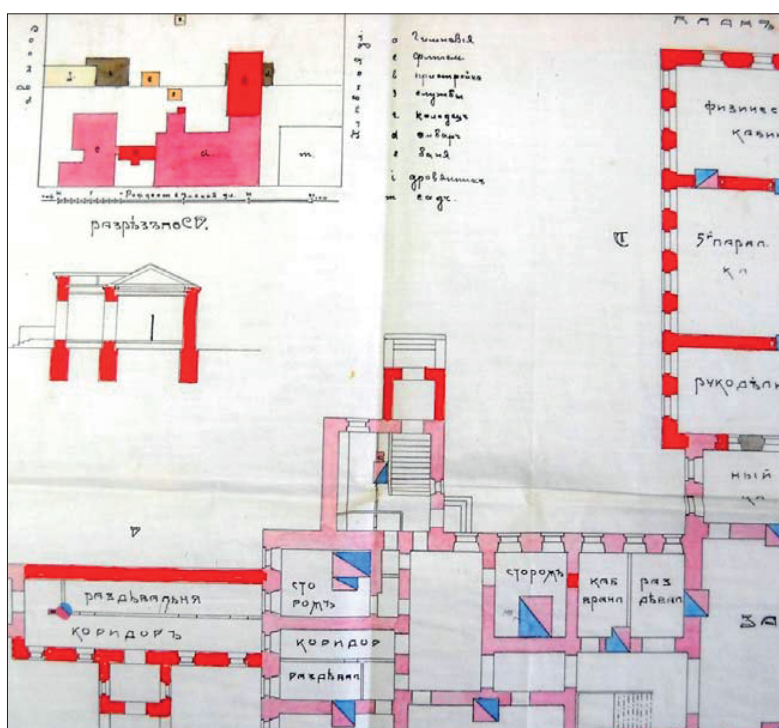
Рис. 3. Проект на пристройку к зданию Слободской женской гимназии. 1909 г. Ф. 583, оп. 532, д. 45
