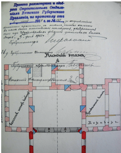
Рис. 10. Проект пристройки к зданию Слободской женской гимназии 1913 г. Ф. 583, оп. 536, ед. хр. 153
