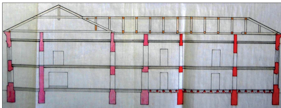
Рис. 6. Проект на пристройку к зданию Слободской женской гимназии. 1909 г. Ф. 583, оп. 532, д. 45
