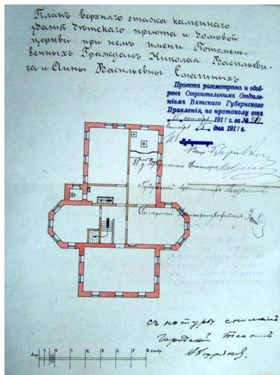
Рис. 8. План верхнего этажа каменного здания детского приюта и домової церкви при немъ имени потомственныхъ гражданъ Н. В. и А. В. Смагиных. 1913 г. [4]
