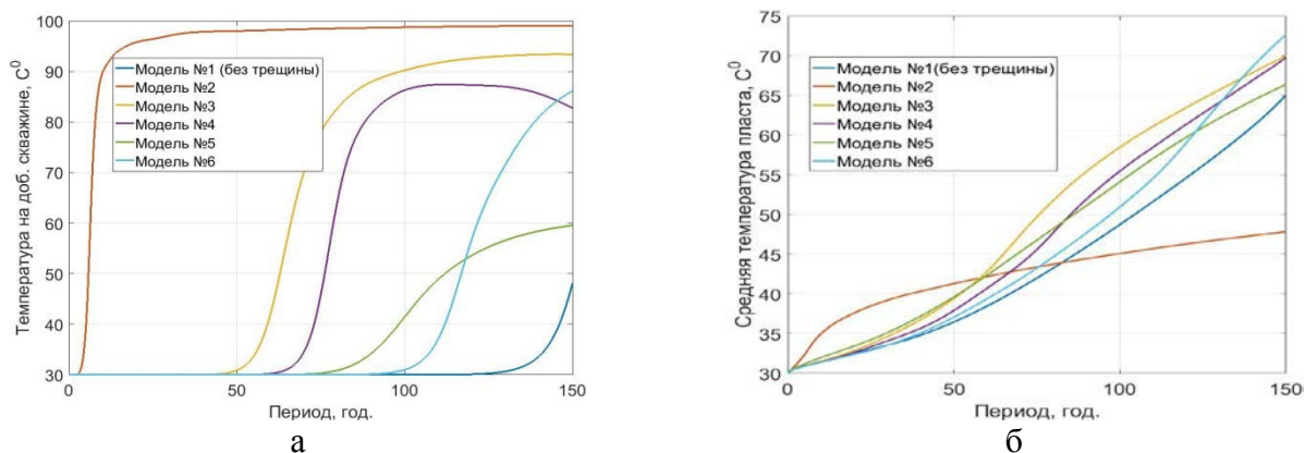
Рис. 10. Динамика изменения температуры для моделей пласта №№1-6: а – температура добываемой жидкости, б – средняя температура пласта
