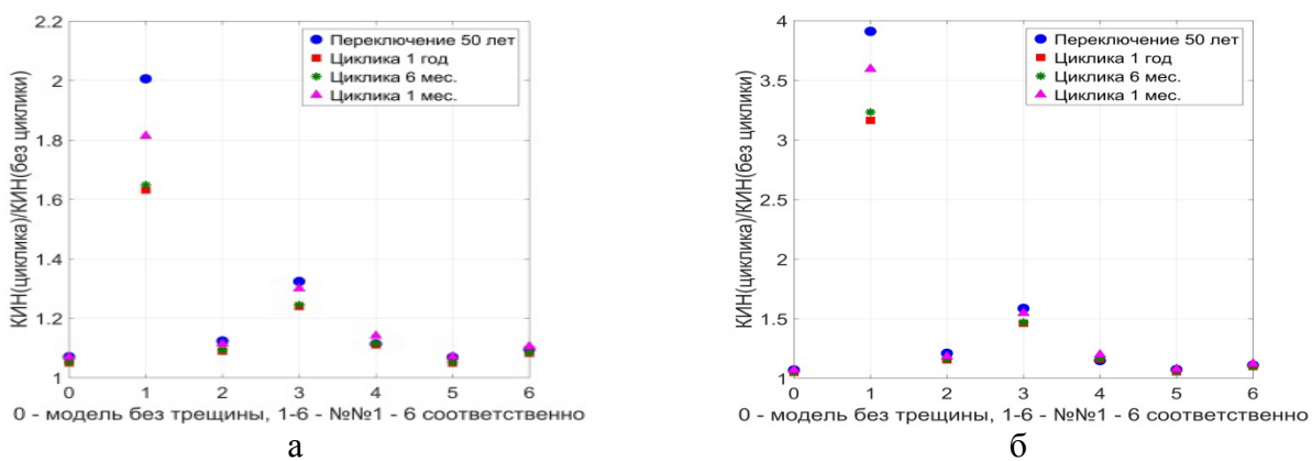
Рис. 4. Отношение значений КИН (нестационарное заводнение) к КИН (стационарное заводнение) в моменты времени, соответствующие достижению предельной обводненности добываемой жидкости 0,97. Проницаемость трещин равна: а – 10^3 мД, б – 10^4 мД
