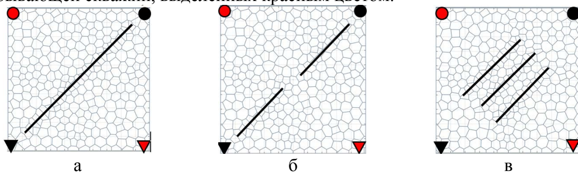
Рис. 1. Различные варианты положения трещин в расчетной области при ориентации трещины 0^\circ относительно главного направления потока жидкости: а – модель №1, б – модель №2, в – модель №3
