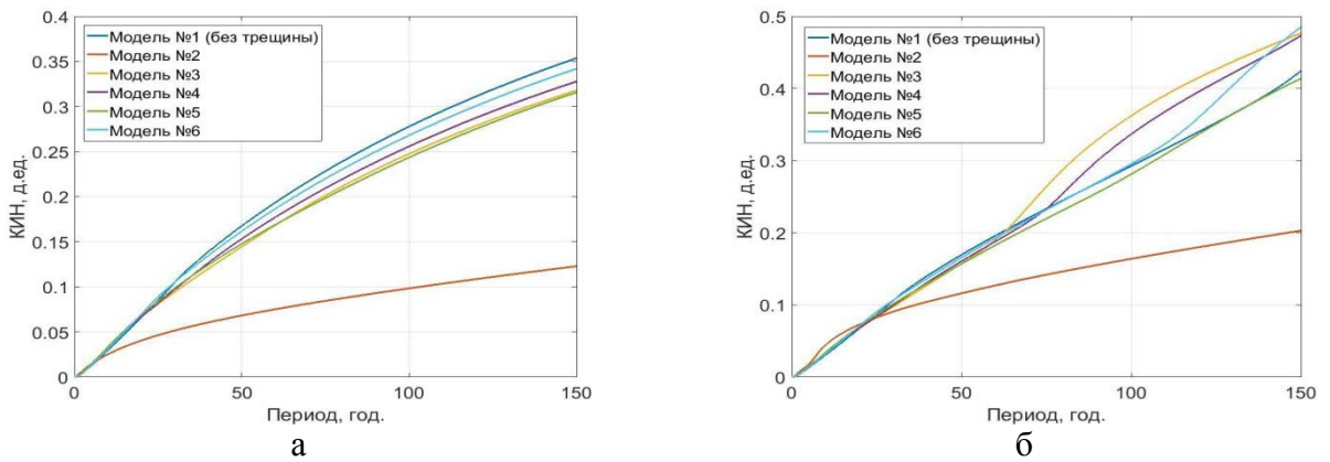
Рис. 8. Зависимости КИИ от времени для моделей пласта №№1-6: а – температура закачиваемой воды – 30°C, б – температура закачиваемой воды – 100°C
