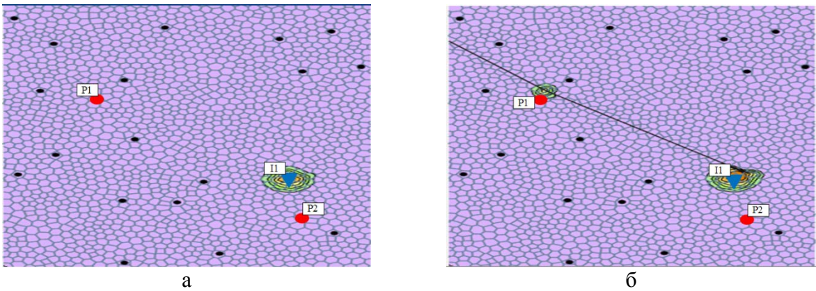
Рис. 13. Поля температур 21.02.2015: а – для модели №1, б – для модели №2
