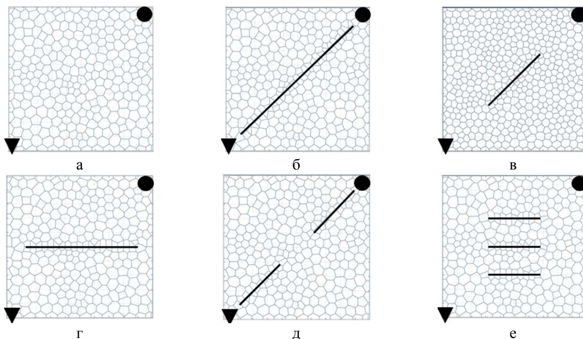
Рис. 7. Синтетические модели пласта: а – модель №1(без трещины), б – модель №2, в – модель №3, г – модель №4, д – модель №5, е – модель №6
