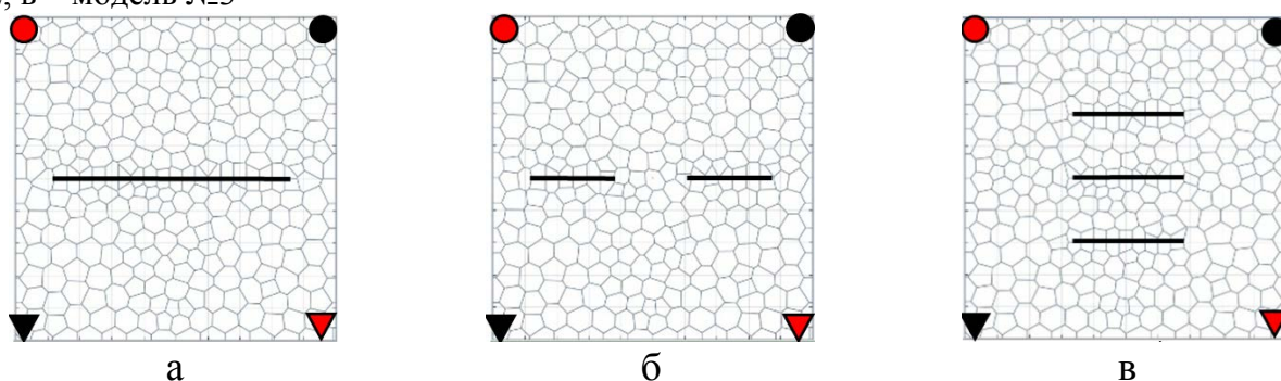
Рис. 2. Различные варианты положения трещин в расчетной области при ориентации трещины 45^\circ относительно главного направления потока жидкости: а – модель №4, б – модель №5, в – модель №6
