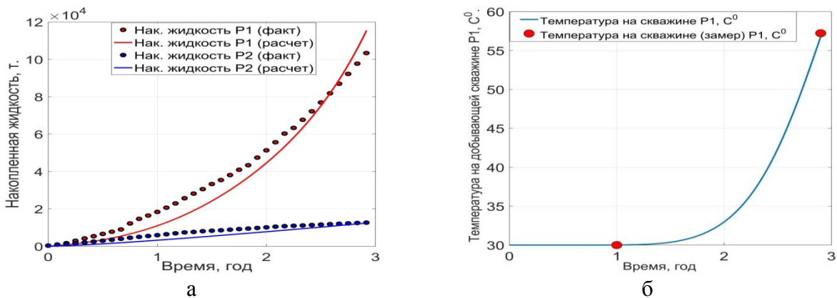
Рис. 14. Сопоставление результатов расчетов с фактическими данными: а – накопленная жидкость скважин P1 и P2 для модели №2, б – температура добываемой жидкости на скважине P1 для модели №2
