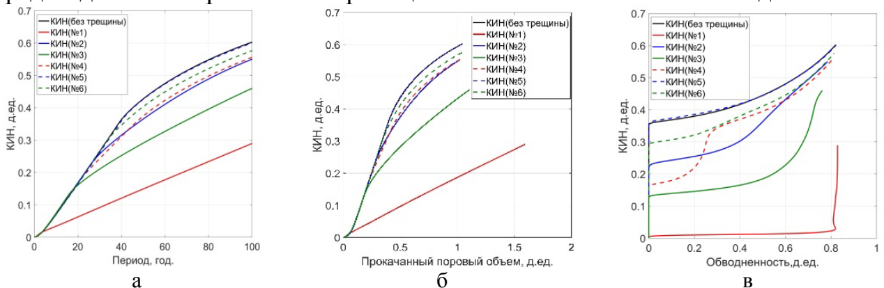
Рис. 3. Зависимости КИН для моделей пласта №№1-6 для случая стационарного заводнения (проницаемость трещин - 10^3 мД): а – от времени, б – от прокачанного порового объема, в – от обводненности
