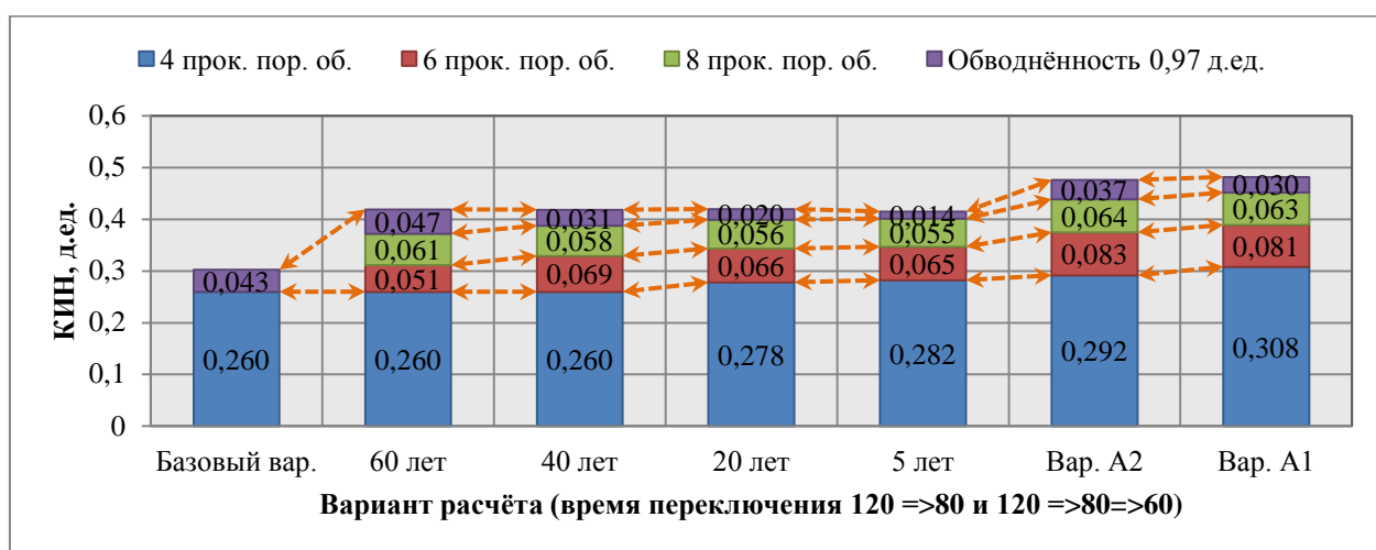
Рис. 5. Значения и изменение КИН для различных вариантов времени снижения темпа закачки воды
