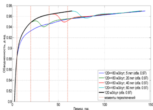
Рис. 6. Зависимость обводненности от времени для \beta_f - 0,1
