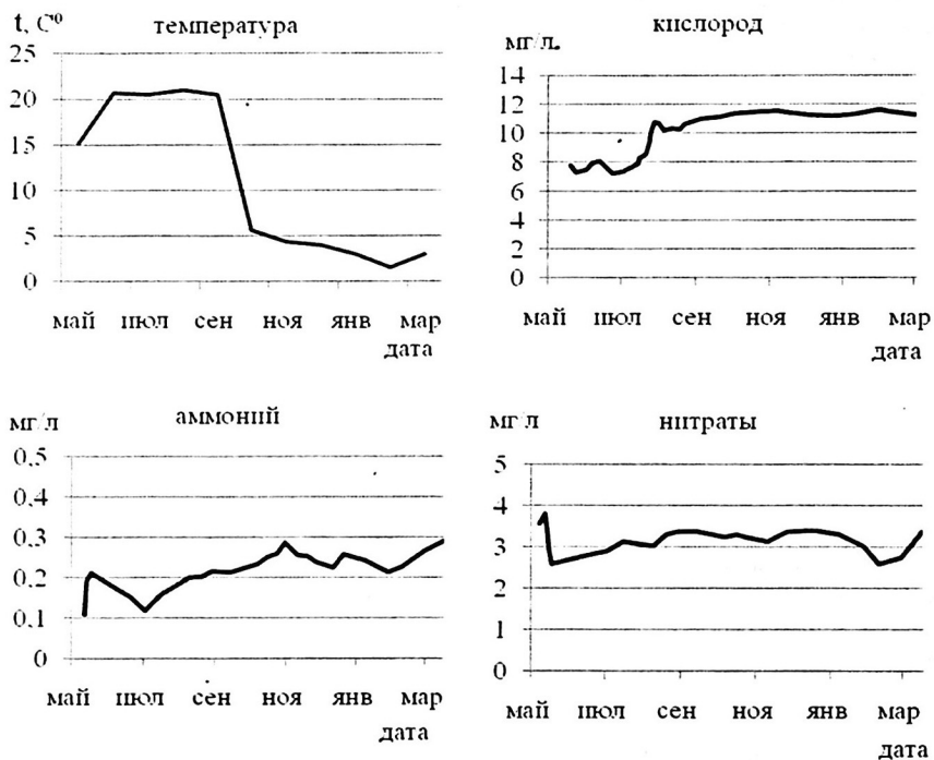
Рис. 1. Динамика некоторых показателей водного режима в УЗВ (2009-10 гг.)
