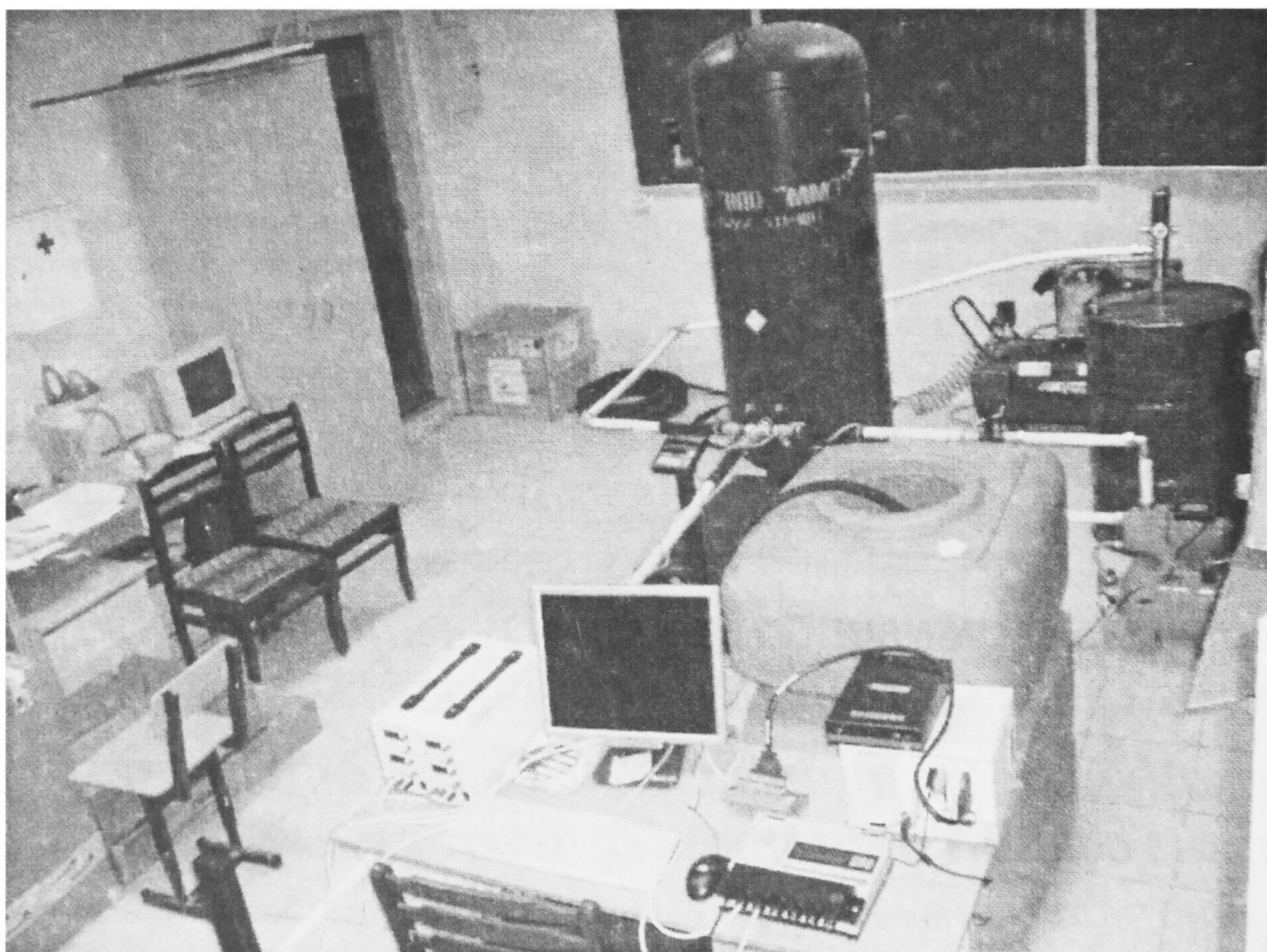
Рис. 1. Стенд многофазных потоков
