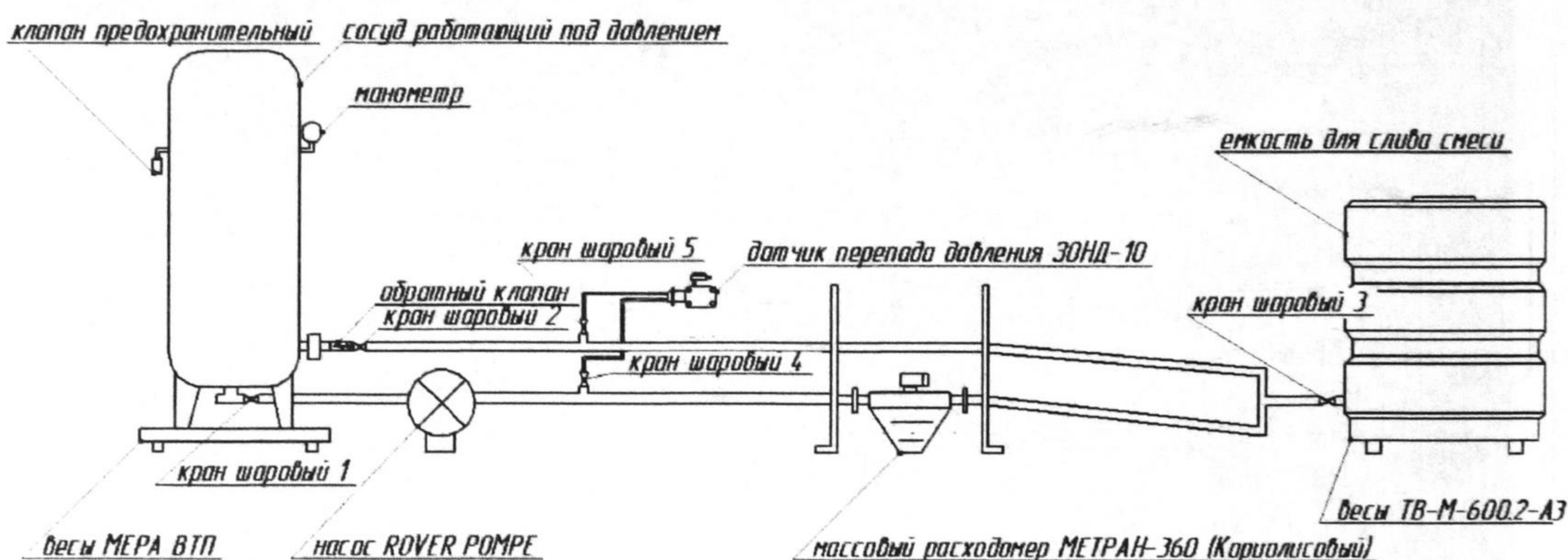
Рис. 3. Линия для поверки расходомеров
