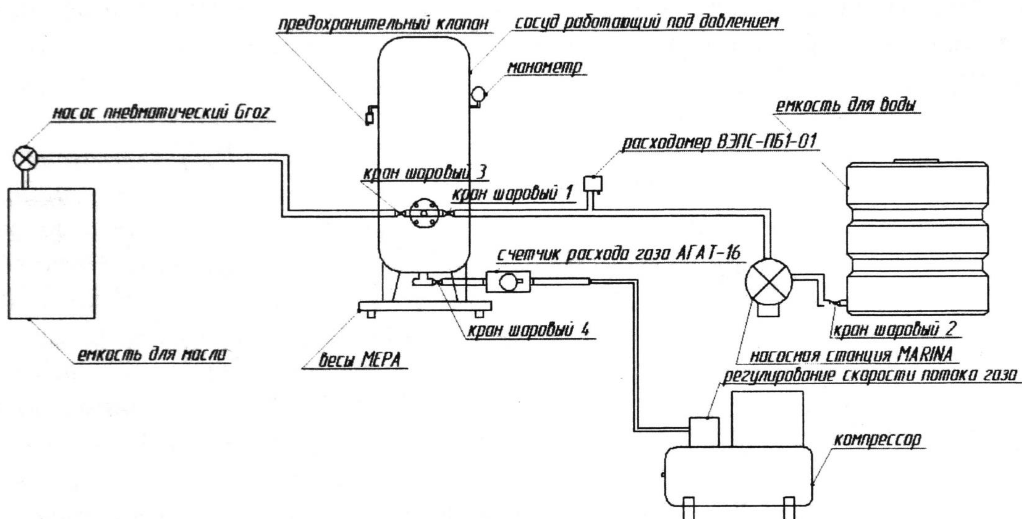
Рис. 2. Установка для приготовления многофазной смеси
