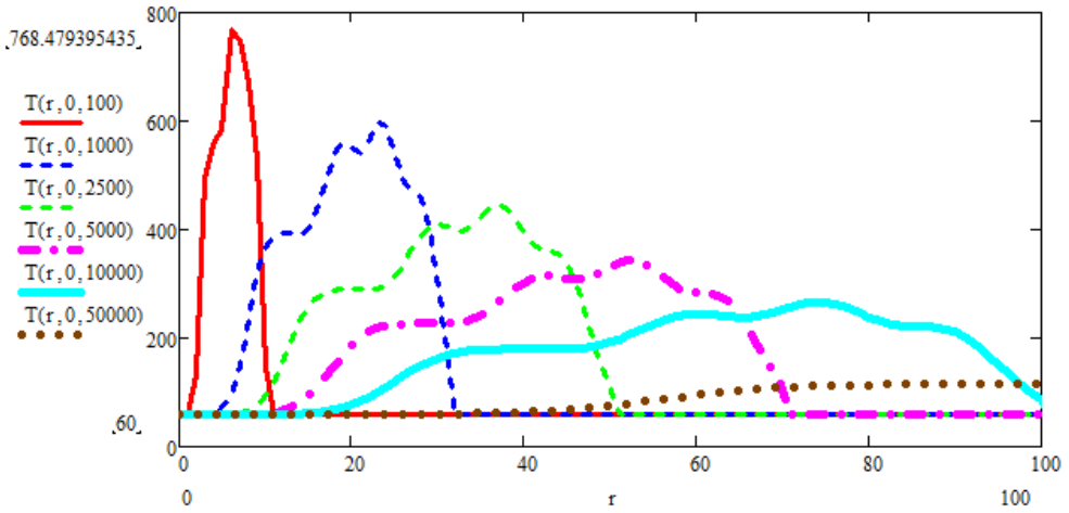
Рис. 6. Динамика изменения профиля температур в пласте от времени. Дебит воздуха: q_b = 60 тыс. \text{м}^3/\text{сут} ; масса топлива в единице объема: z = 13 \text{ кг}/\text{м}^3 ( Pe = 5,87 )
