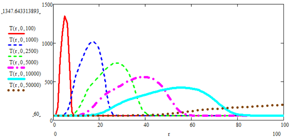
Рис. 7. Динамика изменения профиля температур в пласте от времени. Дебит воздуха: q_b = 60 тыс. \text{м}^3/\text{сут} ; масса топлива в единице объема: z = 24 \text{ кг}/\text{м}^3 ( Pe = 5,87 )
