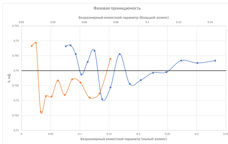
Рис. 4. Фазовая проницаемость
