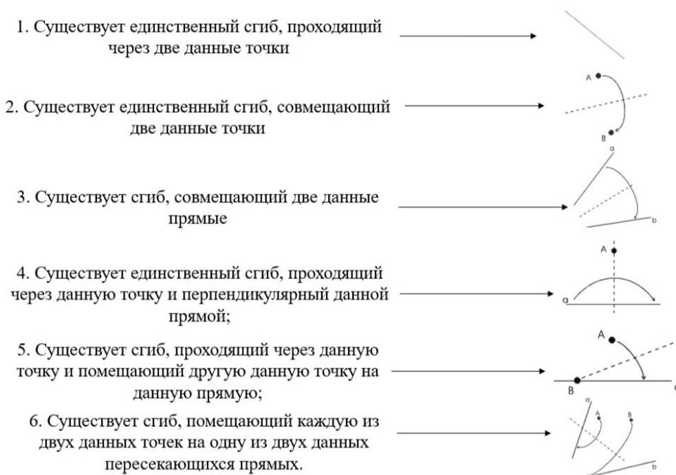
Рис. 2. Аксиомы оригаметрии
