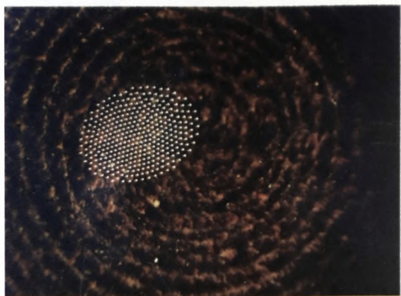
Одна из первых фотографий капельного кластера. На квадратном миллиметре жидкой поверхности может легко поместиться несколько тысяч капелек.
