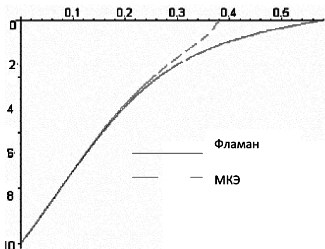
Рис. 3. Вертикальные перемещения x_1 = 0 . Прямоугольник 10*10 (м) сторона 0,1 м
