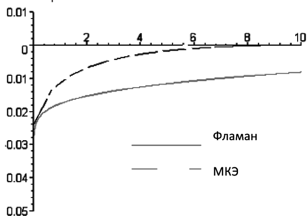
Рис. 4. Осадки для сетки 10*10 (м) со стороной 1 м
