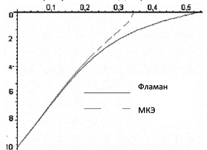
Рис. 2. Вертикальные перемещения x_1 = 0 . Прямоугольник 10 \times 10 (м) сторона 0,7 м
