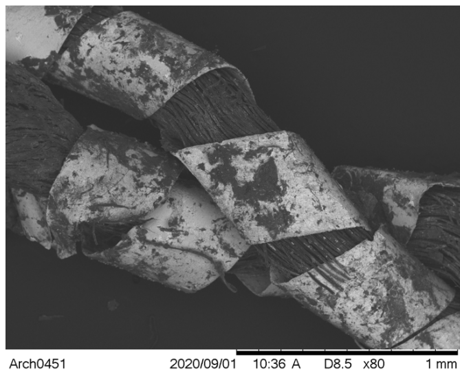
Рис. 6. Металлическое покрытие первого образца золотой нити (80-кратное увеличение)
