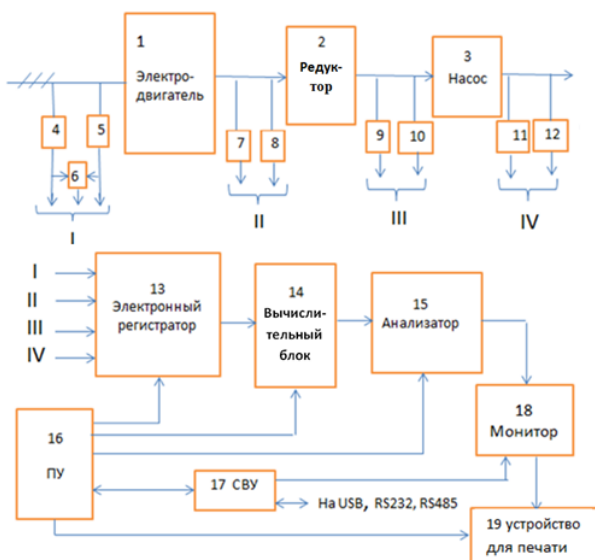
Рис. 1. Структурная схема устройства для диагностики и определения энергоемкости работы насосного агрегата: 1 — электродвигатель; 2 — редуктор; 3 — насос; 4 — измеритель напряжения; 5 — измеритель тока; 6 — измеритель \cos \varphi ; 7 — измеритель крутящего момента; 8 — измеритель скорости вращения; 9 — датчик крутящего момента; 10 — датчик скорости вращения; 11 — измеритель напора; 12 — измеритель расхода; 13 — электронный регистратор; 14 — вычислительный блок; 15 — анализатор; 16 — пульт управления; 17 — система высшего уровня; 18 — монитор; 19 — устройство для печати; I, II, III, IV — группы соединений
