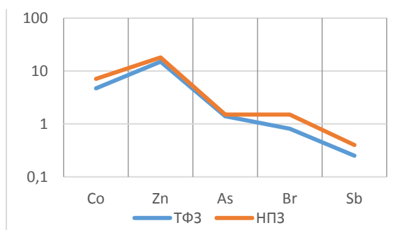
Рис. 4. Содержание химических элементов в горизонте A1 почвы территории расположения Антипинского нефтеперерабатывающего завода в сравнении с Тюменским федеральным заказником (мг/кг, логарифмическая шкала)
