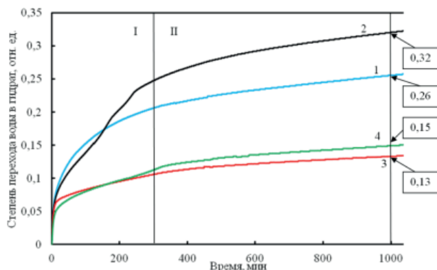
Рис. 7. Изменение степени перехода воды в гидрат метана в дисперсном льду (1), ЗВДС с добавлением АН 1,5 масс. % (2) и 0,15 масс. % (3) и ЗВДС с добавлением ГК 1 масс. % (4). Давление начала эксперимента 5 МПа, температура 272,2 К. Дисперсность образцов 80–140 мкм
